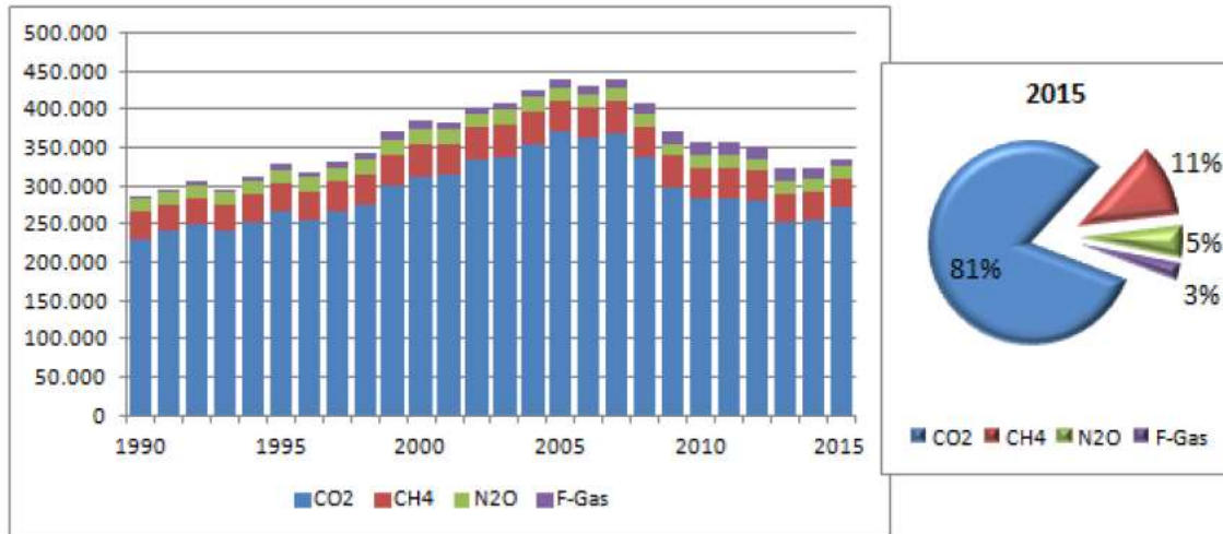
Figura 109. Distribución anual das emisións de GEI por gas e detalle para o ano 2015
