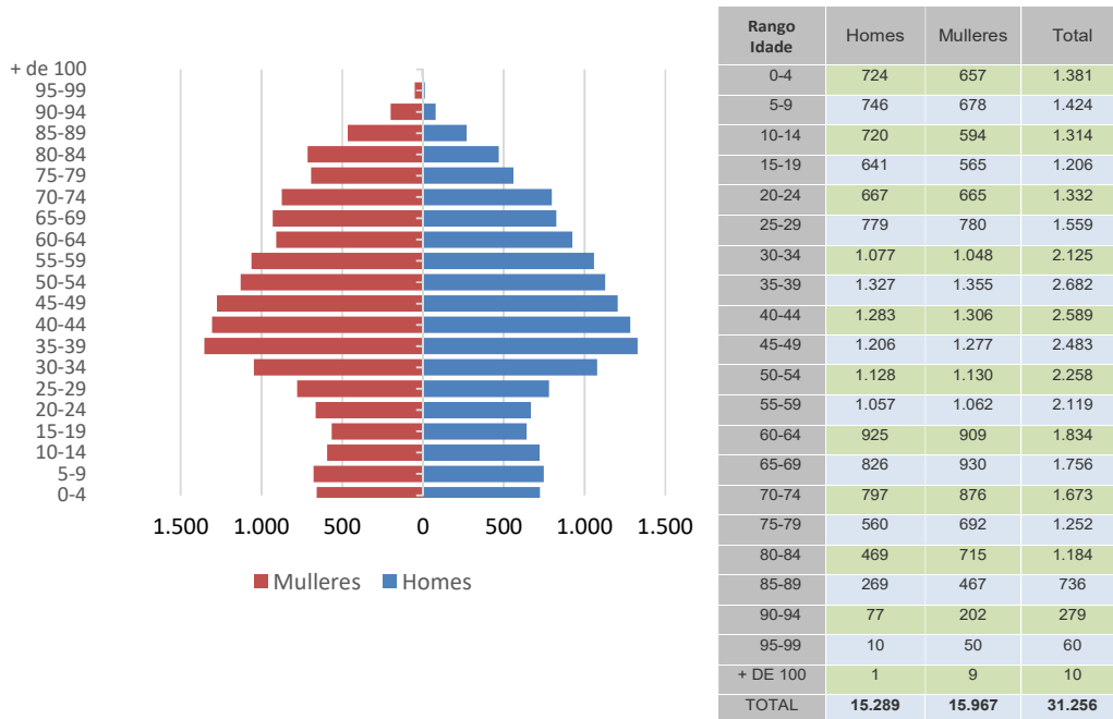
Figura 7. Pirámide poboacional
