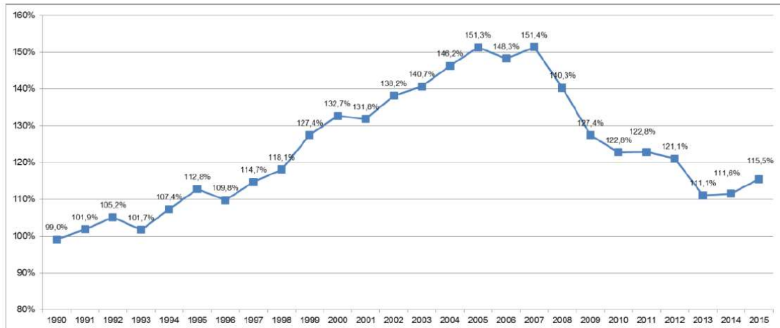
Figura 106. Evolución das emisións de GEI tomando como referencia o primeiro ano da serie (1990)
