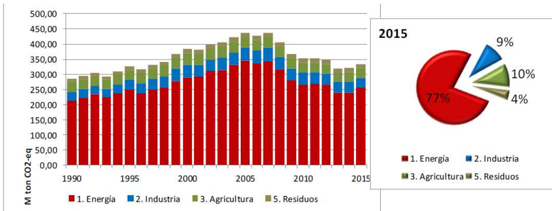
Figura 108. Distribución anual das emisións de GEI por grupo de actividade e detalle para o ano 2015
